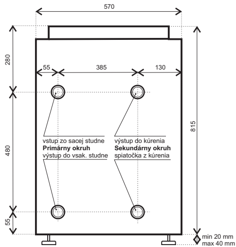
Zadný pohľad
