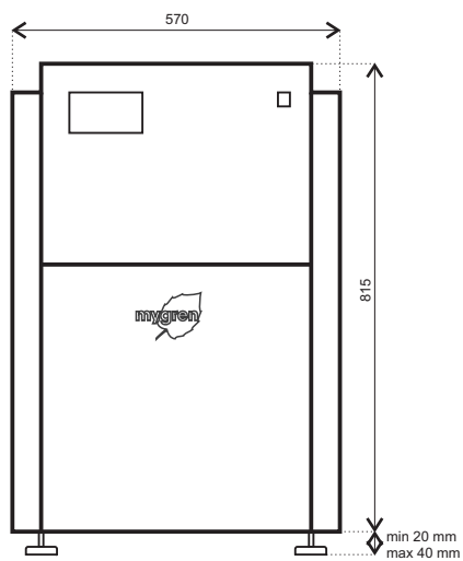
Čelný pohľad
