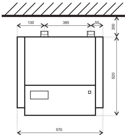
Pohľad zvrchu
