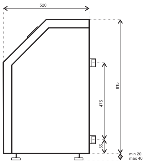
Bočný pohľad
